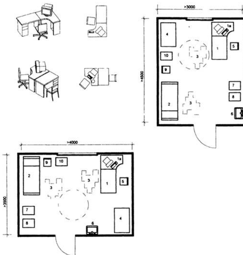
Блокировка стола врача со столом для персонального компьютера
