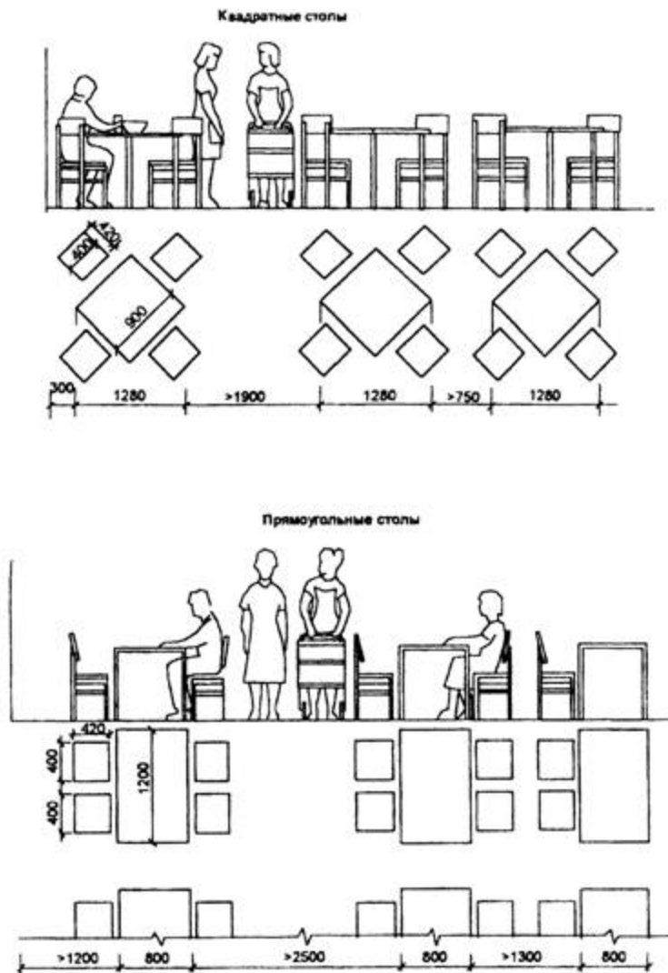
Рис. 17 Места в залах общественного питания
