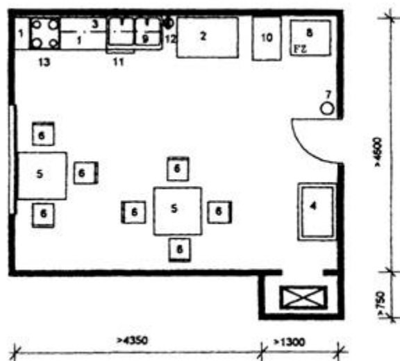
Рис. 13 Общая комната-столовая и кухня
